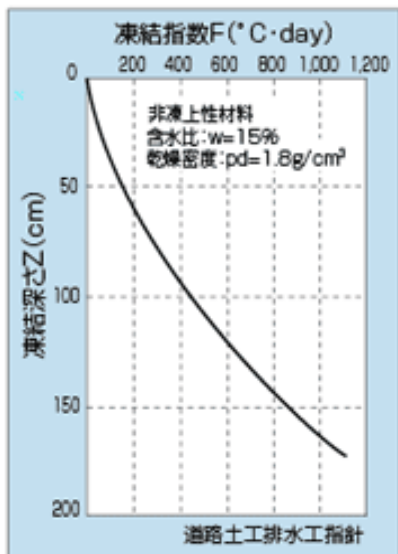
図-1 凍結深さと凍結指数との関係の例
